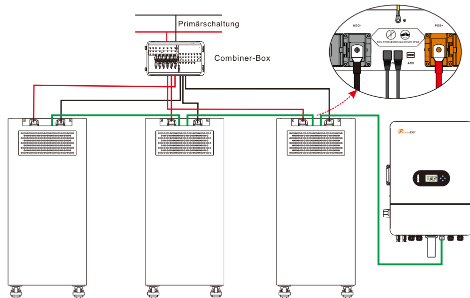
Abbildung 1: Die Parallelschaltung von drei Akkupacks
